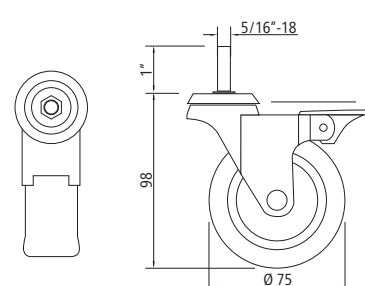
75121 23 702 Dimensions
