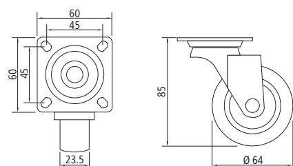
75123 23 010 Dimensions
