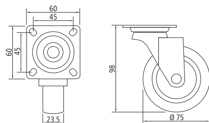
75123 23 012 Dimensions
