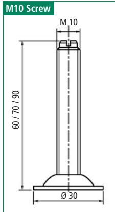
M10 Screw
