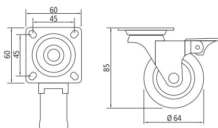
75121 23 011 Dimensions
