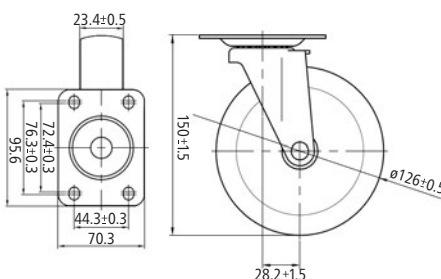
75123 12 007 Dimensions
