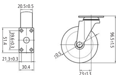
75123 12 004 Dimensions
