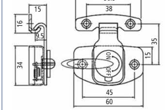
Dimensions
