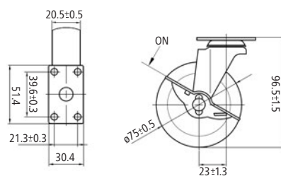
75121 12 000 Dimensions
