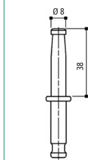
Socket Stem
