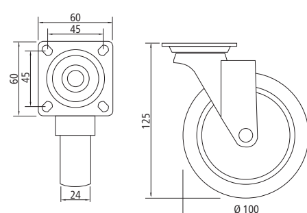
75123 23 008 Dimensions
