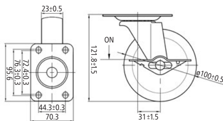
75121 12 002 Dimensions
