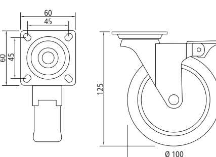
75121 23 009 Dimensions
