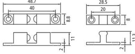
Dimensions
