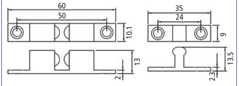
Dimensions
