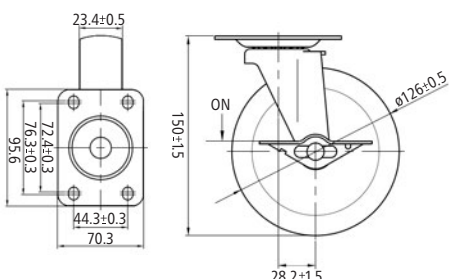
75121 12 002 Dimensions
