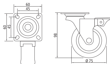
75121 23 014 Dimensions
