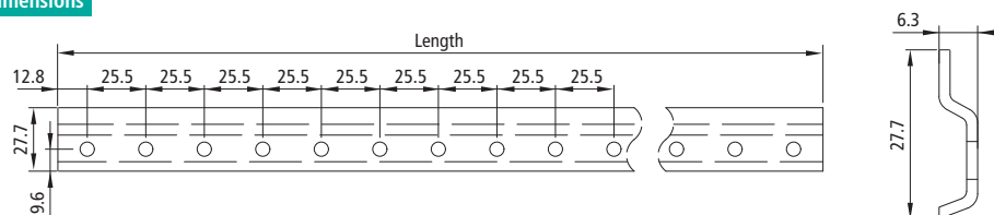
Dimensions
